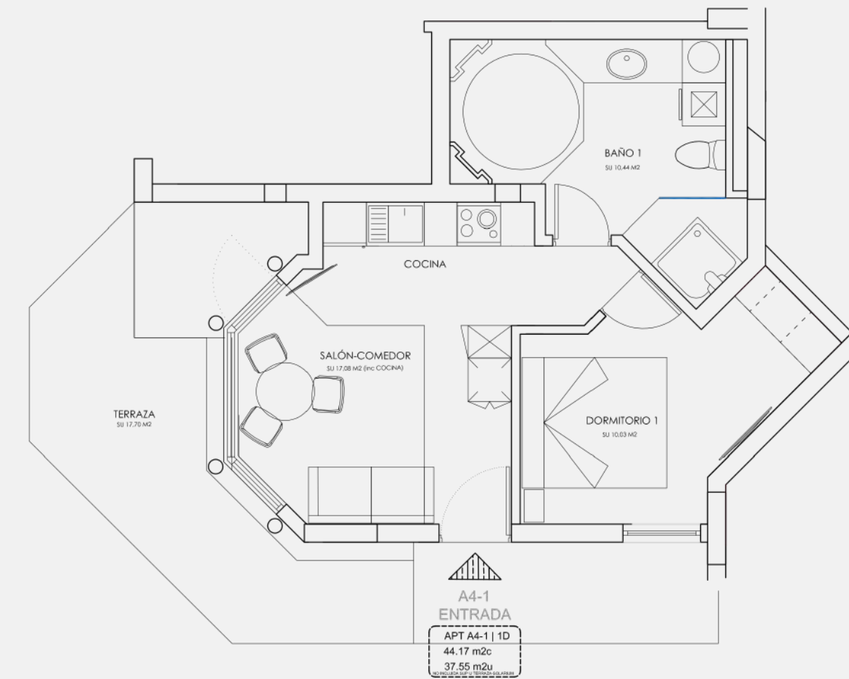
APARTAMENTO A4-1 TIPO 3
