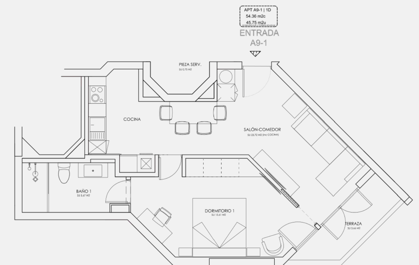
APARTAMENTO A9-1 TIPO 8
