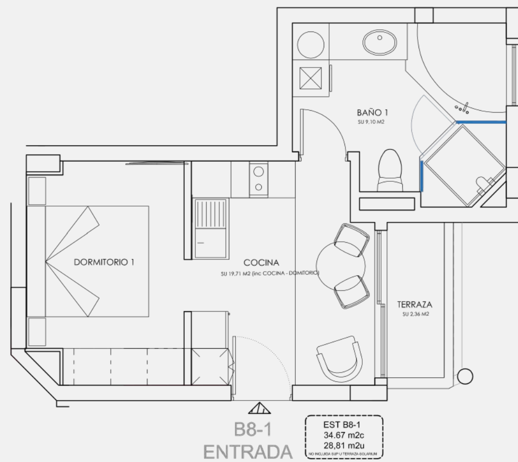
APARTAMENTO B8-1 TIPO 5
