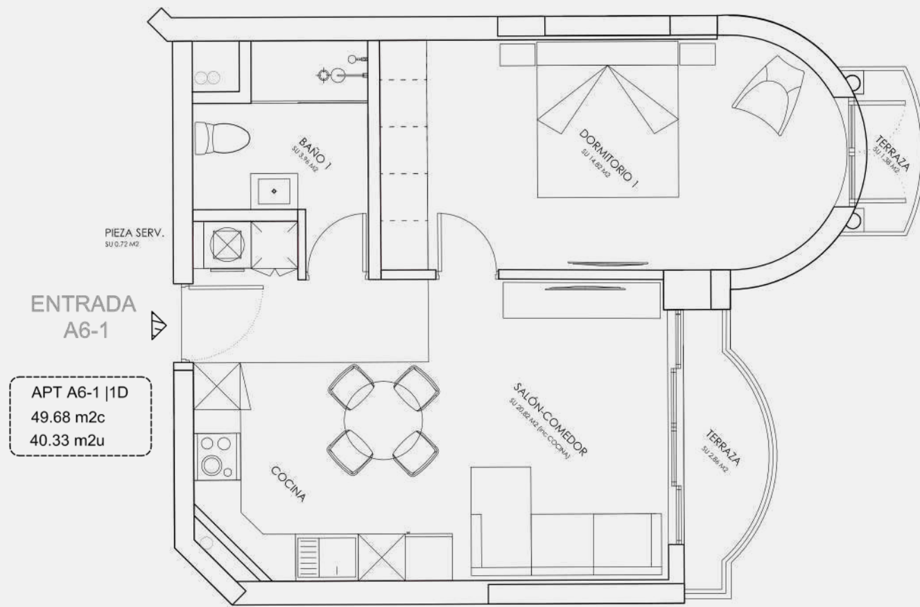
APARTAMENTO A6-1 TIPO 1
